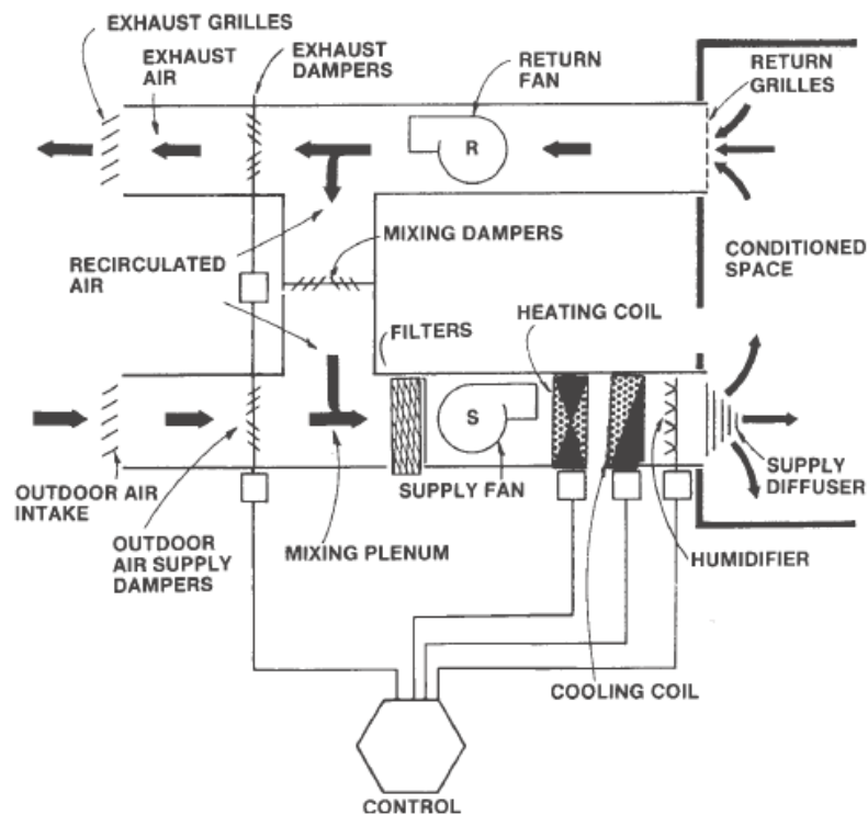
Figura 6 - Componentes de um sistema de ventilação mecânica.
