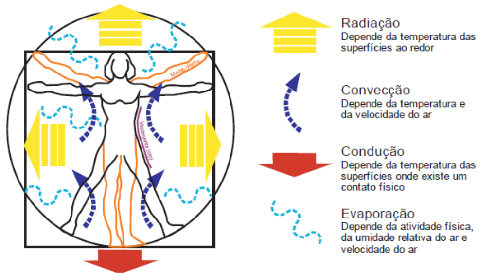
Figura 2 - Representação esquemática da fisiologia humana e a trocas térmicas.
