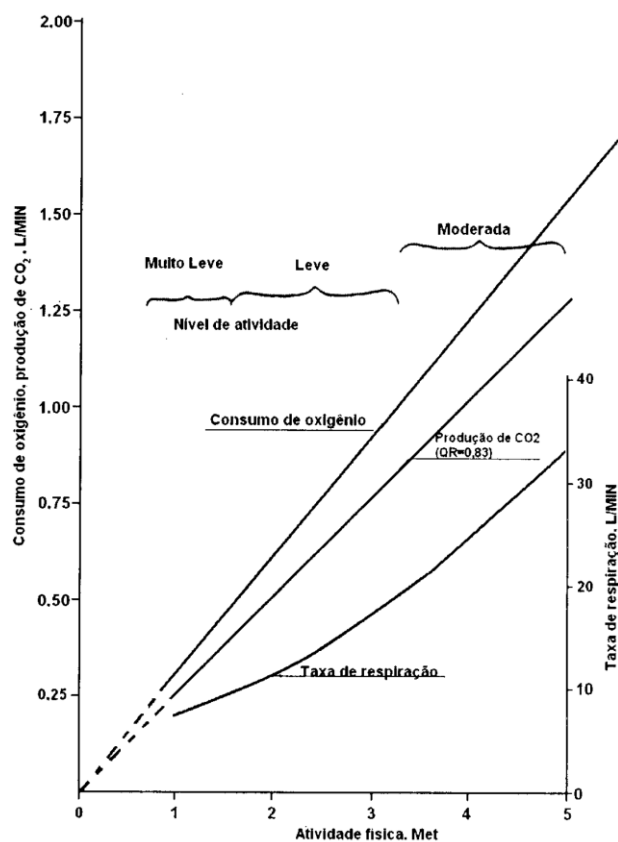
Figura 5 - Taxa de respiração, consumo de oxigênio e produção de \text{CO}_2 em função do metabolismo.
